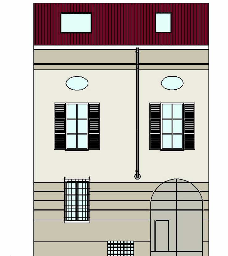
FRONTE
